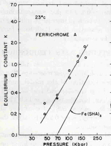
Fig. 6. \text{Ln}K vs. \text{Ln}P for ferrichrome A.
